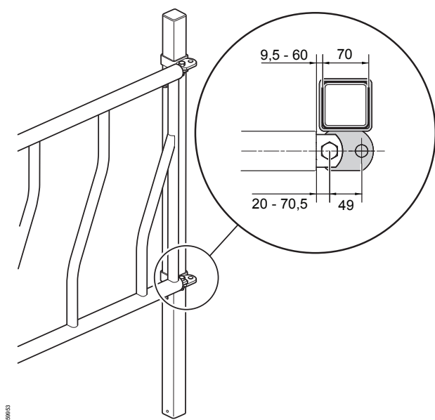
Fig. 5: Fôrfront DS-W festet foran på en 70 x 70-stolpe.
