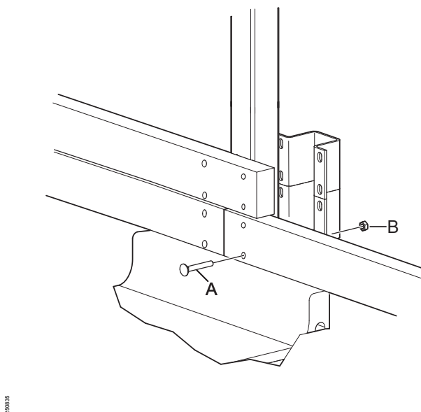
Fig. 16: Montere treplanke
