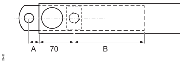
Fig. 6: Justerbart jern.
