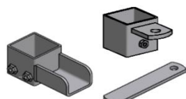
691202-210 (sæt) 2" fanggitre, højre/venstre. Fladjern i top og uskål midt i bund.
