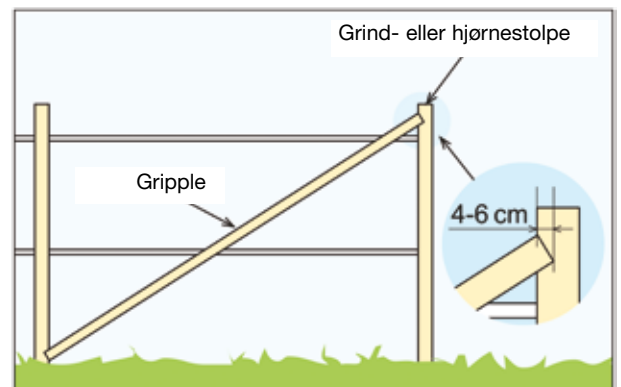
Bilde 4. Alternativ 2 Hjørne-/grindforsterkning med støtte. OBS! Det er viktig å lage et 4-6 cm stort uttak i stolpene slik at festet blir sterkt for støttene.
