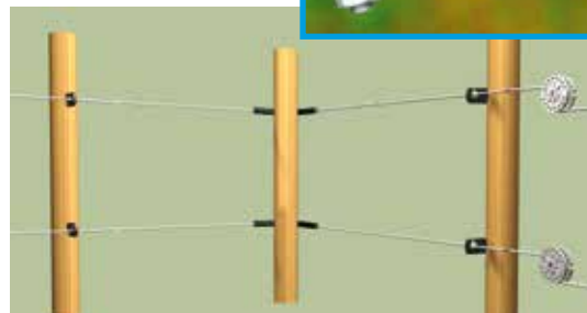
Bilde 5 og 6. Isolatorrør eller eggisolator i hjørnene.
