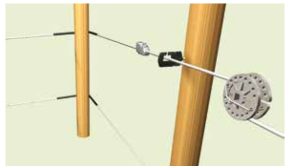
Bilde 19. Trådspstrammere gjør det enkelt å holde tråden stram.
