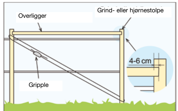
Bilde 3. Alternativ 1 Hjørne-/grindforsterkning med parallelogram. OBS! Det er viktig å lage et 4-6 cm stort uttak i stolpene slik at overliggeren får et sterkt feste.
